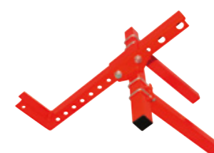
KIT DI MONTAG- GIO PER SUP- PORTO CUBICO, GANCIO TRAINO E SUPPORTO SPONDA (PICK- UP)
